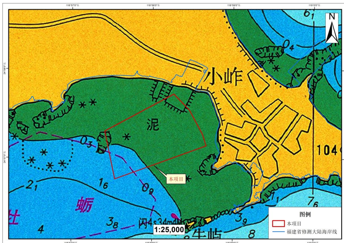
图 1.4-2 项目区水深地形图
