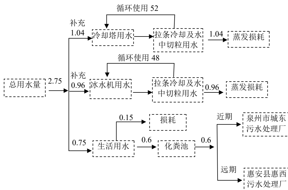
图 2.7-1 项目水平衡图（单位：t/d）
