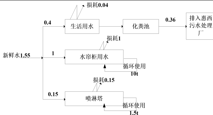
图 2-1 本项目水平衡图
