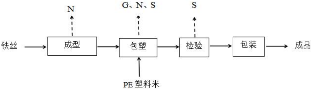
图 2-4 铁制日用品(衣架)生产工艺流程及产污环节
