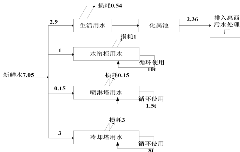
图 2-2 全厂水平衡图
