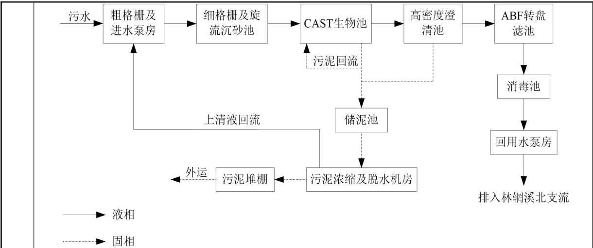
图 4-1 惠西污水处理厂工艺流程图
