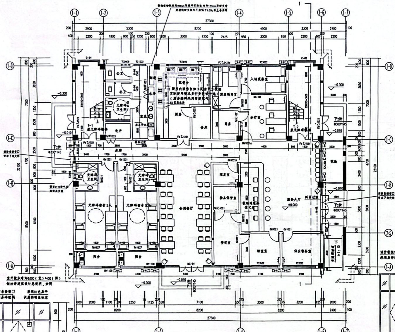
一层平面图 1:100 本层建筑面积: 543.97 平方米, 占地面积: 543.97 平方米 总建筑面积: 1620.11 平方米, 本层高度: 16 米, 层高: 5.0 米
